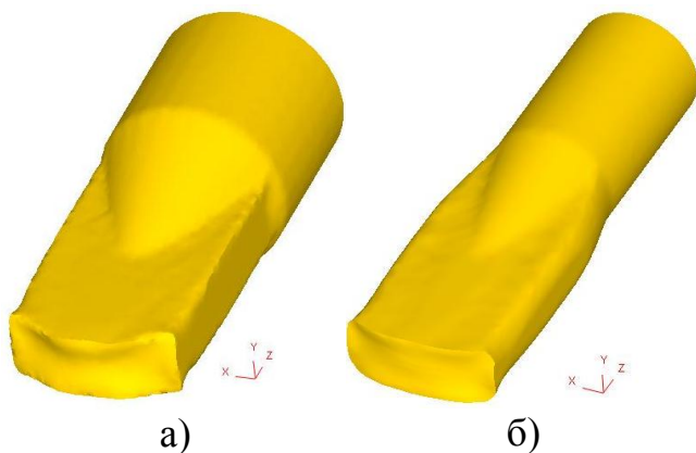
Рис. 2. Сдеформированные заготовки для традиционного выдавливания (а) и выдавливания с раздачей (б).
