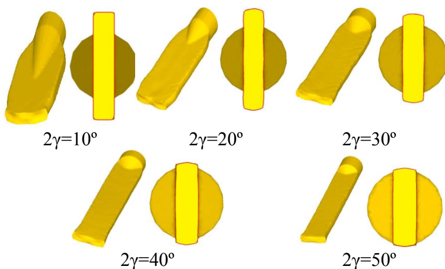
Рис. 7. Влияние угла конуса матрицы 2\gamma на заполнение профиля.
