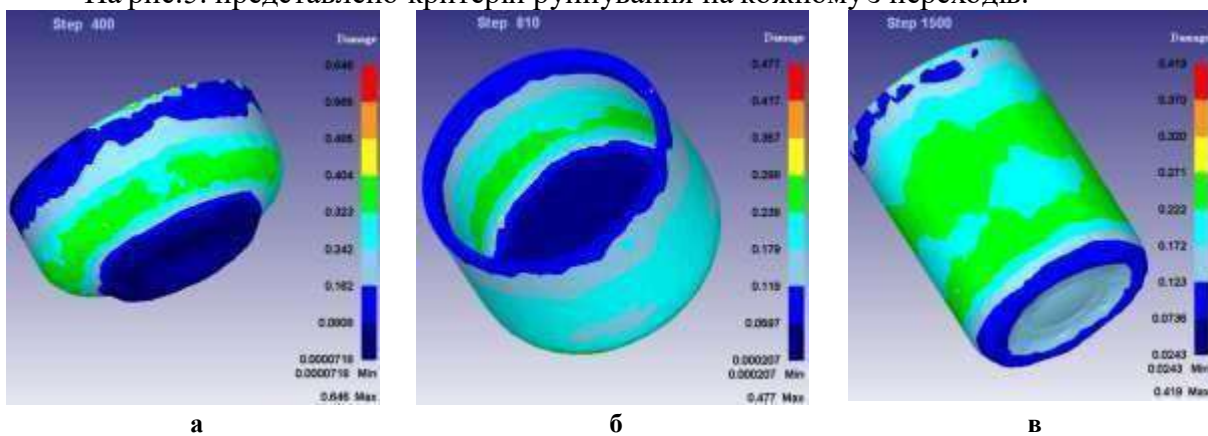
Рис.5. Критерій руйнування:
