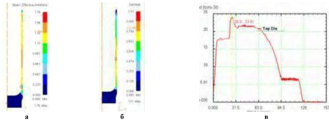
Рис. 6. Результати моделювання витягування з потоншенням одночасно через дві матриці з використанням пластичної моделі матеріалу: а - розподіл інтенсивності деформації; б - картина розподілу значень критерію руйнування Normalized C&L; в - діаграма зусилля
