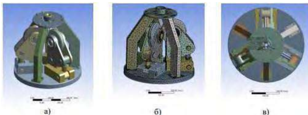
Рис. 1 - а) CAD-модель пристрою; б) сітка кінцевих елементів; в) силове навантаження на ролики
