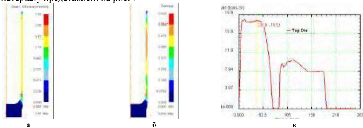
Рис. 7. Результати моделювання витягування з потоншенням послідовно через дві матриці з використанням пружно-пластичної моделі матеріалу: а - розподіл інтенсивності деформації; б - картина розподілу значень критерію руйнування Normalized C&L; в - діаграма зусилля
