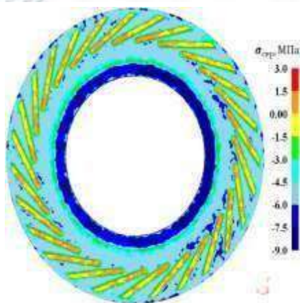
Рис. 4 – Розподіл середніх напружень \sigma_{ср} по об'єму деформованого викову моноколеса
