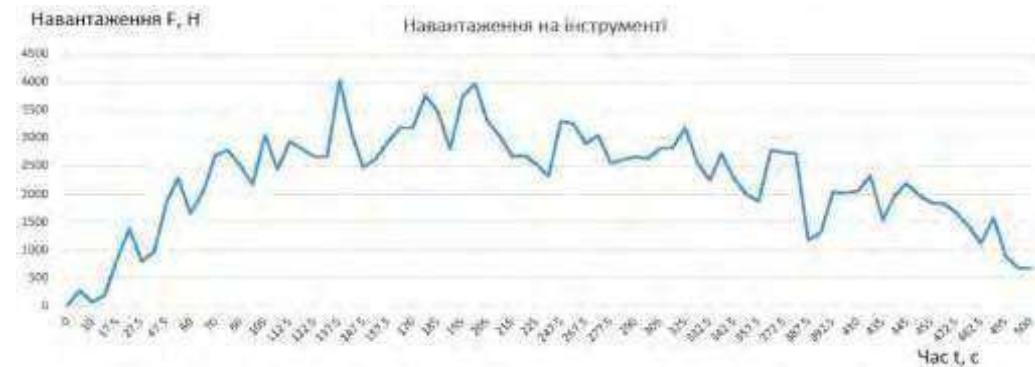
Рис. 5. Навантаження на інструменті по осі X та Y
