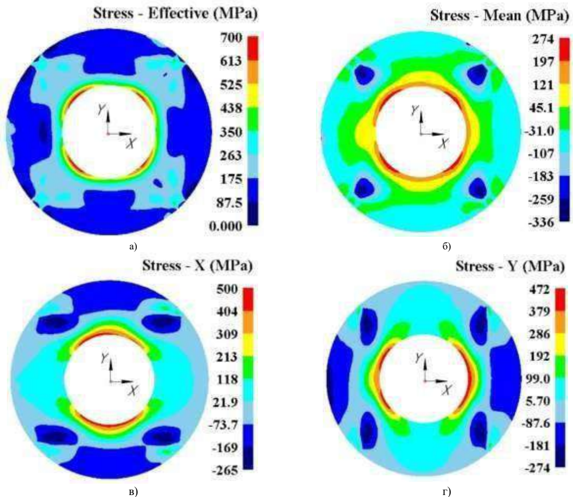
а – інтенсивність напружень \sigma ; б – середні напруження \sigma_{\text{сер}} ; в – напруження \sigma_x ; г – напруження \sigma_y
