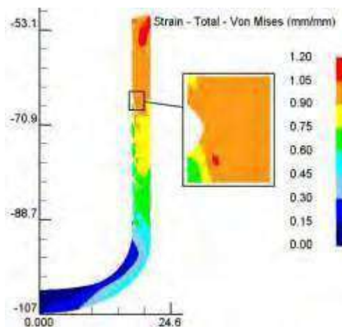
Рис. 8. Розподіл інтенсивності деформації в об'ємі zdeформованої заготовки
