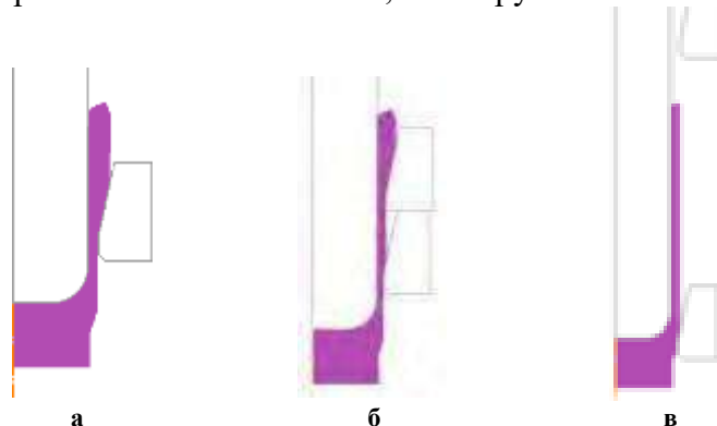
Рис. 1. Схеми витягування з потоншенням:
