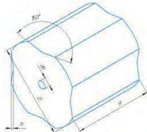
Рис. 1. 3D-модель профільованої заготовки на чотирипроменевий переріз
