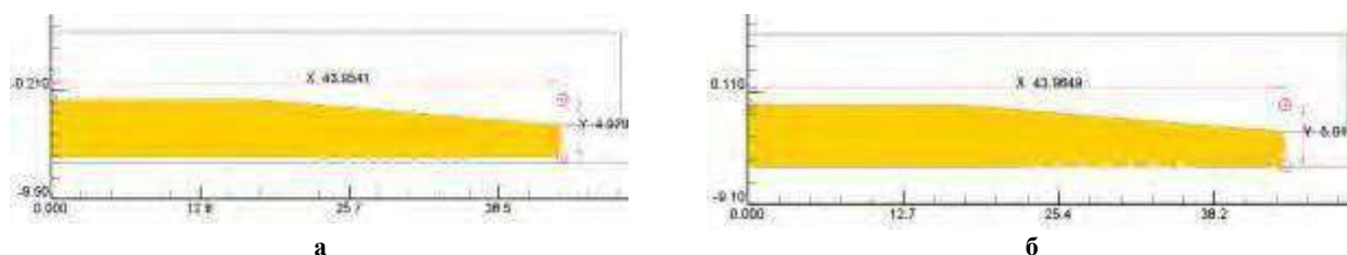
Рис. 5. Розрахункова схема процесу карбування концентраторів на заготовці: а) у вихідному положенні; б) у кінцевому положенні
