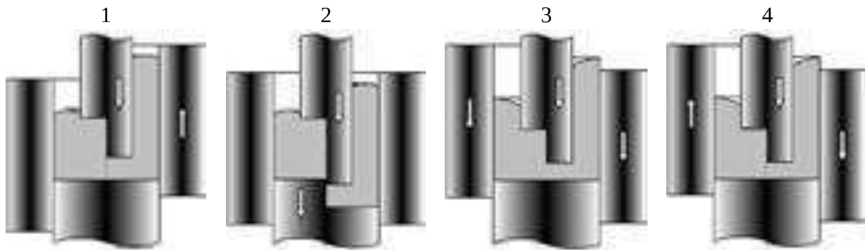
Рис. 1. Способи застосування сил контактної тертя у процесах видавлювання порожнистих деталей
