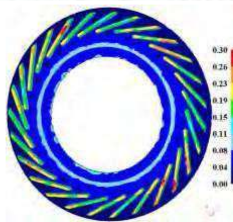
Рис. 5 – Розподіл коефіцієнта використання ресурсу пластичності по об'єму деформованого викову моноколеса
