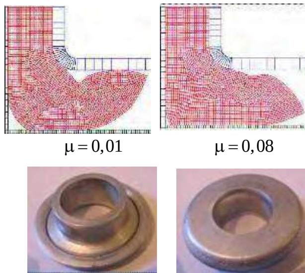
Рис. 4. Спотворення форми фланця при мінімальних силах контактного тертя
