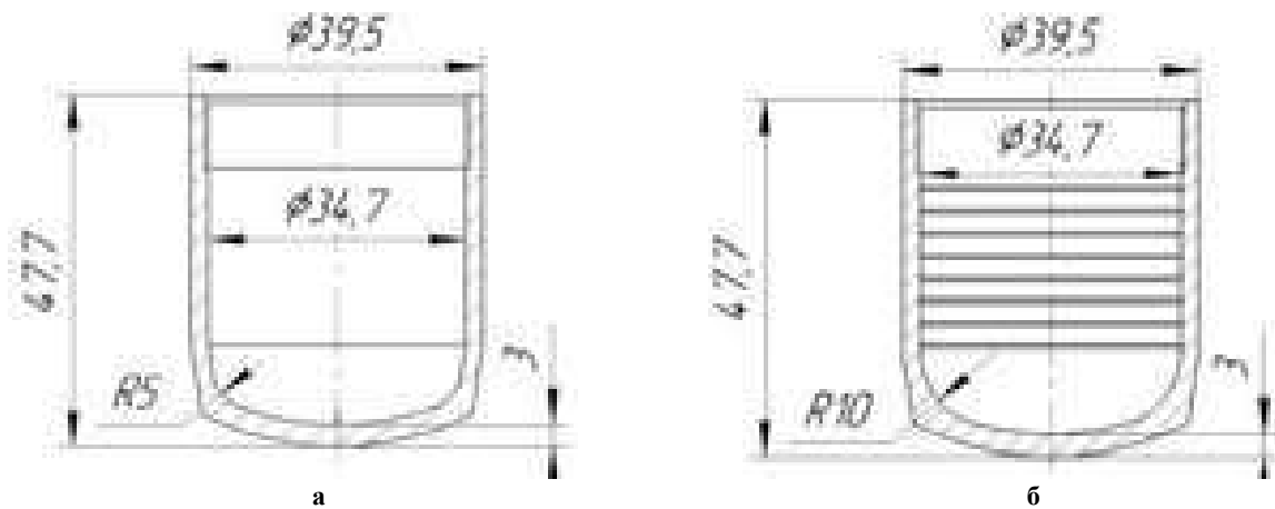
Рис. 1. Ескізи корпусів
