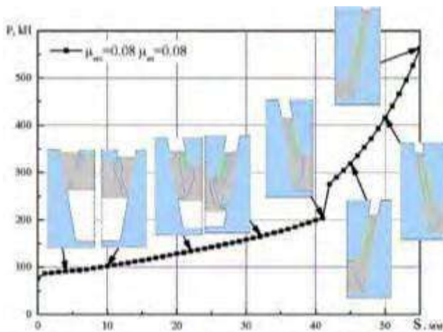
Рис. 3. Характер зміни сили видавлювання Р по ходу пуансону S
