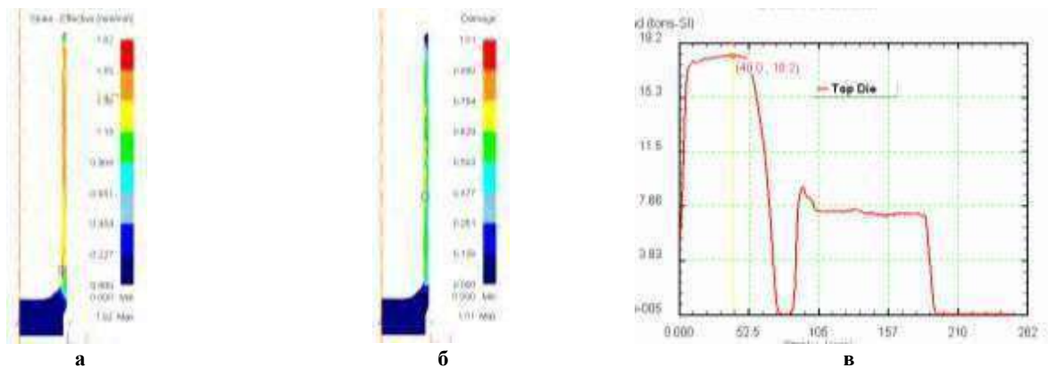
Рис. 8. Результати моделювання витягування з потоншенням послідовно через дві матриці з використанням пластичної моделі матеріалу: а - розподіл інтенсивності деформації; б - картина розподілу значень критерію руйнування Normalized C&L; в - діаграма зусилля
