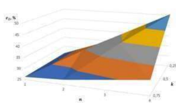
Рис. 4. Гранична поверхня залежності пластичності матеріалу від термомеханічної обробки та кількості переходів.
