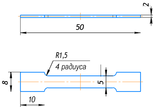
Рис. 1. Креслення зразка
