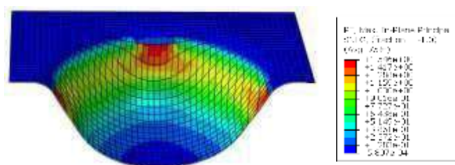
Рис 10. Розподіл максимальних пластичних деформацій
