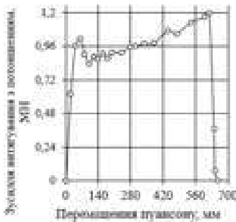
Рис. 4. Залежність зусилля витягування від переміщення пуансону
