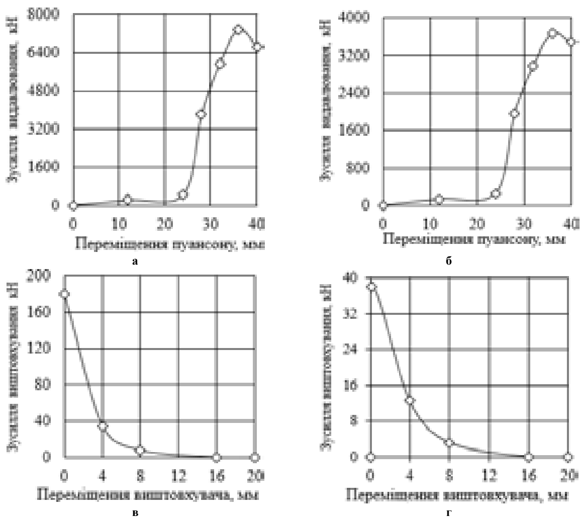
Рис. 2. Силіє режимі видавлювання: а - залежність зусилля видавлювання від переміщення пуансону (заготовка T=700^{\circ}\text{C} ); б - залежність зусилля видавлювання від переміщення пуансону (заготовка T=1000^{\circ}\text{C} ); в - залежність зусилля виштовхування від переміщення виштовхувача ( T=700^{\circ}\text{C} ); в - залежність зусилля виштовхування від переміщення виштовхувача ( T=1000^{\circ}\text{C} )
