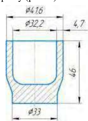
Рис. 2. Порожниста заготовка
