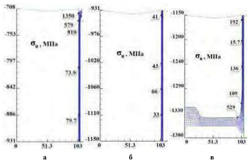
Рис. 5. Розподіли нормальних напружень \sigma_n : а – у верхній частині біля матриці, б – по середині, в- в донній частині
