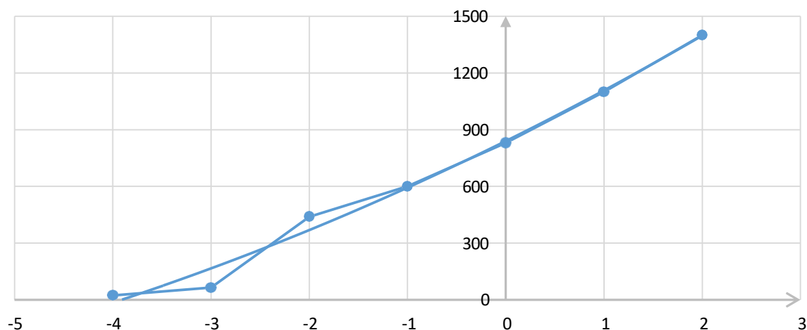
Залежність зусилля деформування P (тс) від логарифму швидкості деформування \log v
