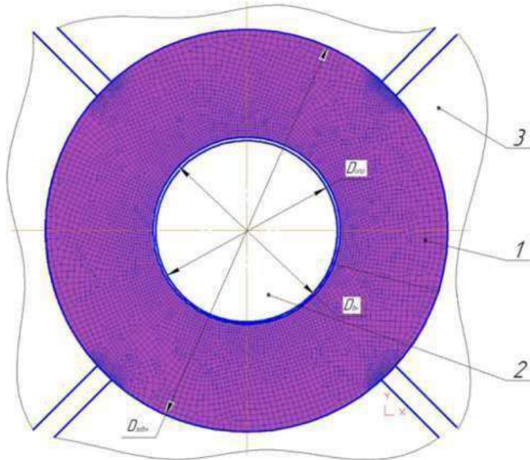
Рис.1 – схема процесу радіального обтиску бойками: 1 – заготовка; 2 – оправка; 3 – бойок
