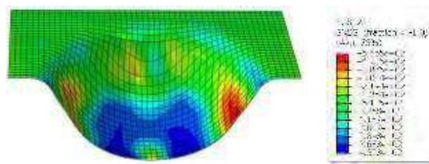
Рис 9. Розподіл напружень \sigma_x
