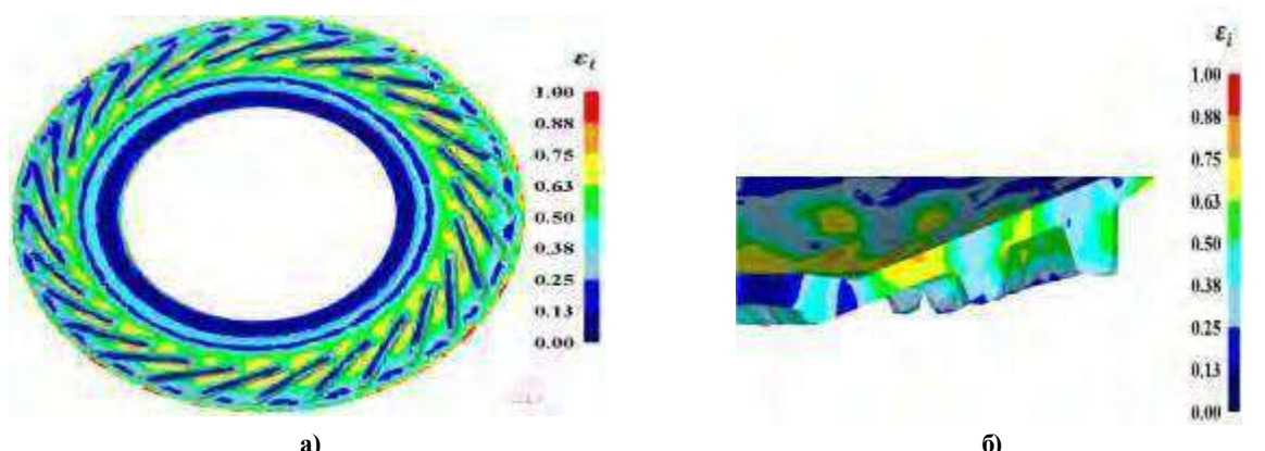
Рис. 2. – Розподіл інтенсивності деформацій \epsilon_i в zdeформованому викові моноколеса: а – по всьому об'єму заготовки, б – в характерному перерізі області пера лопатки
