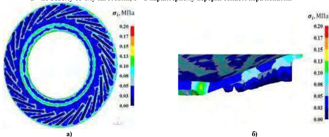
Рис. 3. – Розподіл інтенсивності напружень \sigma_i в zdeформованому викові моноколеса: а – по всьому об'єму заготовки, б – в характерному перерізі області пера лопатки
