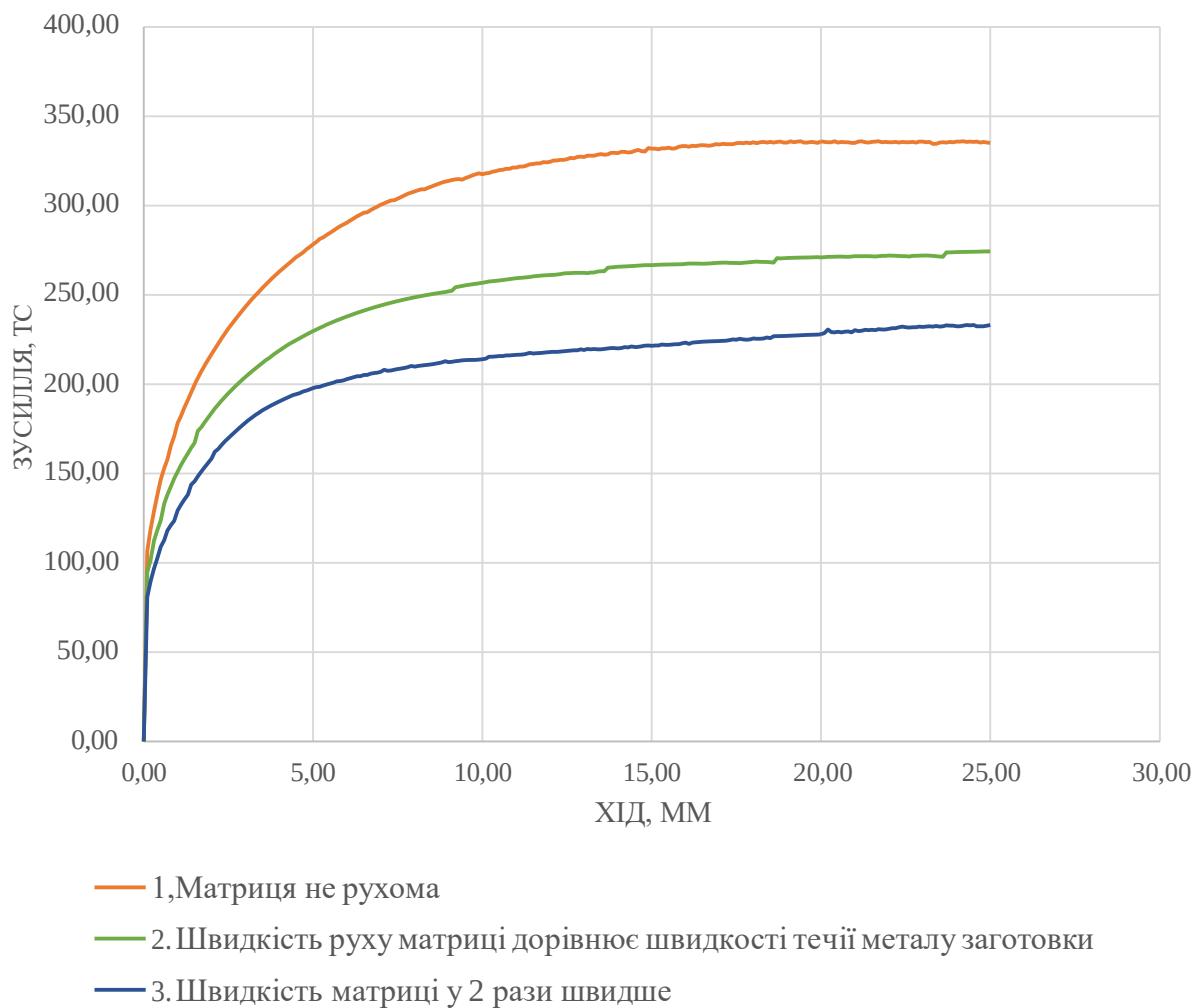
Рис.3 Графік залежності зусилля від ходу при прямому видавлюванні.
